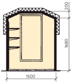
Ristlõige
