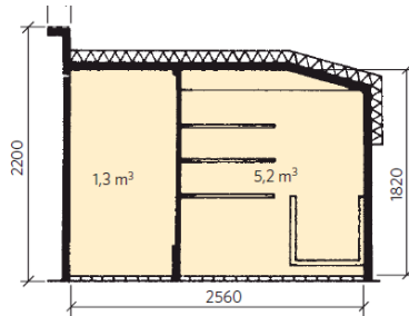
Pikilõige
