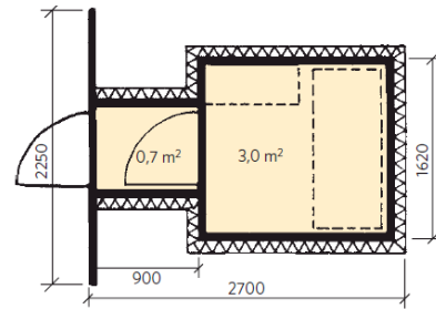
Põhjajoonis
